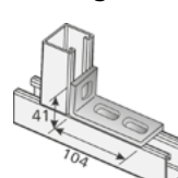
Anschlusswinkel 41 mit Langloch
