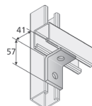
Anschlussverbinder 41 kurz mit Rundloch
