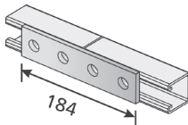
Schienenverbinder 41-F4
