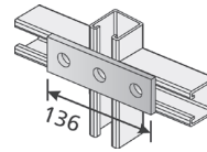
Schienenverbinder 41-F3
