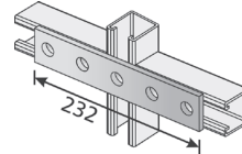
Schienenverbinder 41-F5
