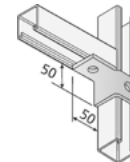
Verbindungswinkel 41 L
