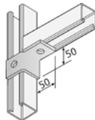
Verbindungswinkel 41 R
