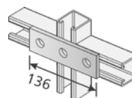
Schienenverbinder 41-F3
