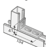
Anschlusswinkel 41 mit Langloch
