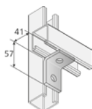
Anschlussverbinder 41 kurz mit Rundloch
